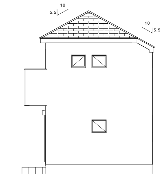
東 EastFacing Elevation
